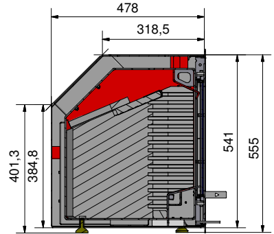
A-A ( 0,12 : 1 )
