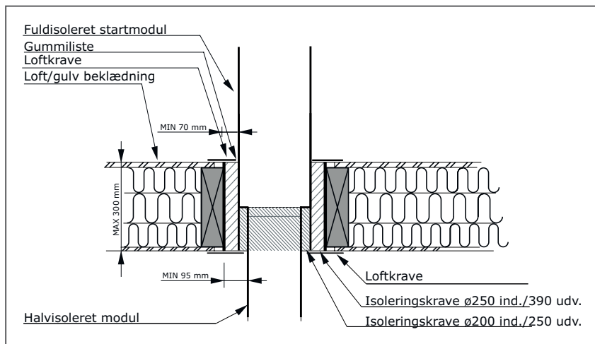
FIG. 1 - Gennemføring i loft/etageadskillelse med skjult overgang
