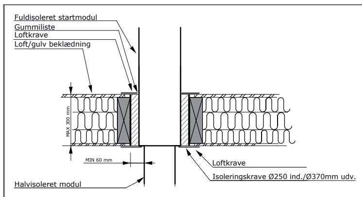
FIG. 2 - Gennemføring i loft/etageadskillelse med skjult overgang
