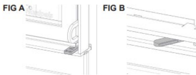
A. Optændingsspjæld B. Luftspjæld Trykket ind= Lukket Venstre = Lukket Trukket ud = Åbent Højre = Åbent
