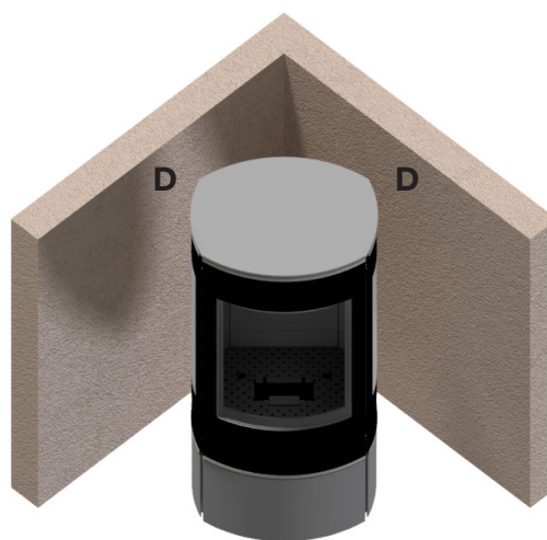
Hjørneinstallation
