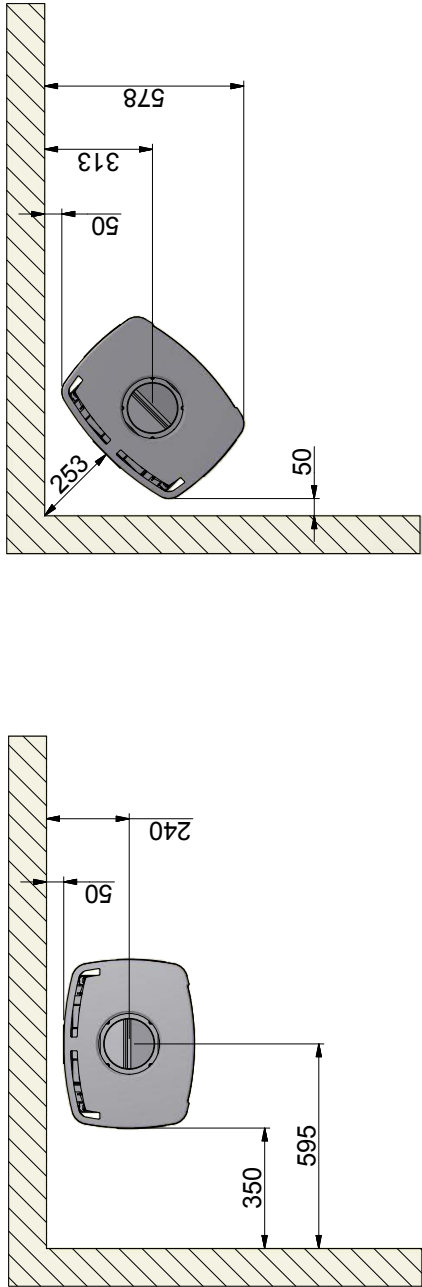
Min. afstand til brændbart materiale (uden sideglas)
