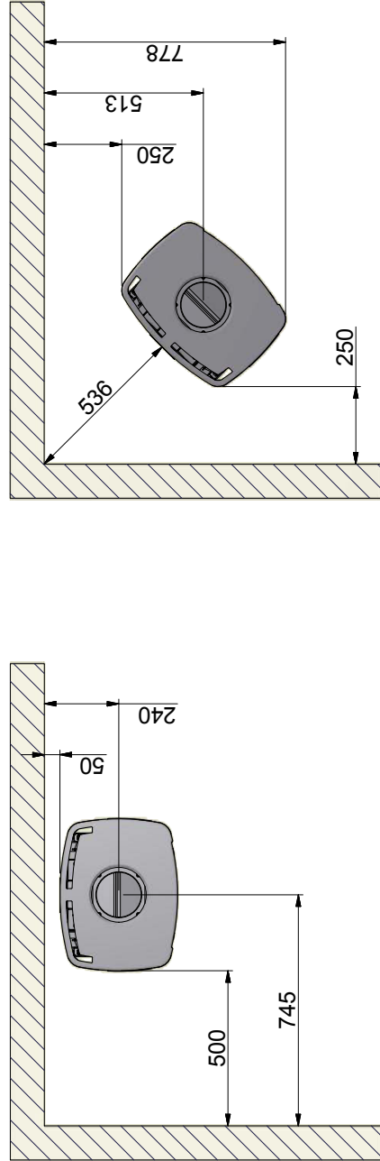
Min. afstand til brændbart materiale (med sideglas)
