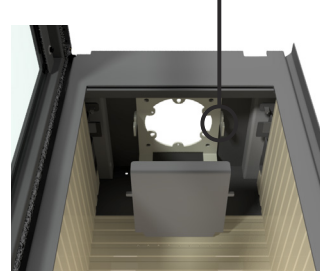
Røgchikanen ved at løfte den op og frem så den kommer fri af fikseringerne
